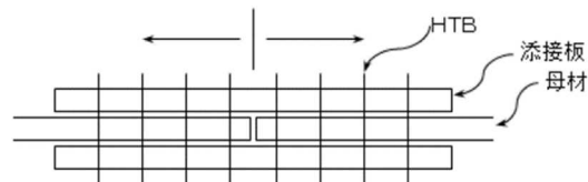
図3-1-1 ボルト締め付け順序
