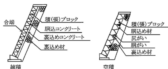
図3-1-4 コンクリートブロック工
