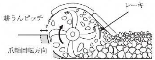
アップカットロータリーによる耕うん
