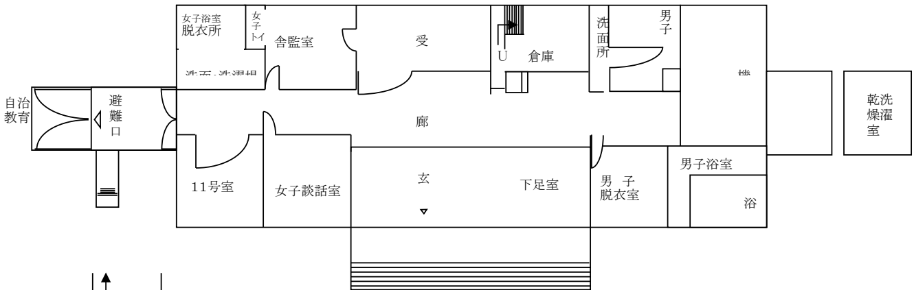
1階平面図
