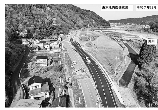
山本地内整備状況 (日本海側を望む)
