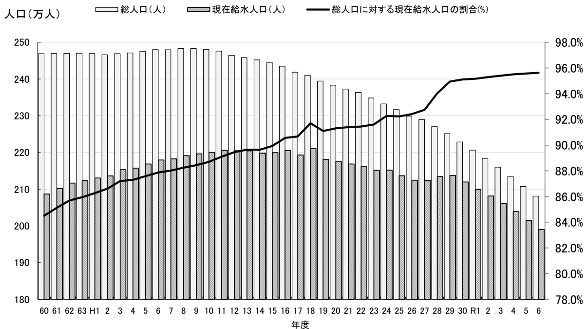
上水道の普及状況の推移
