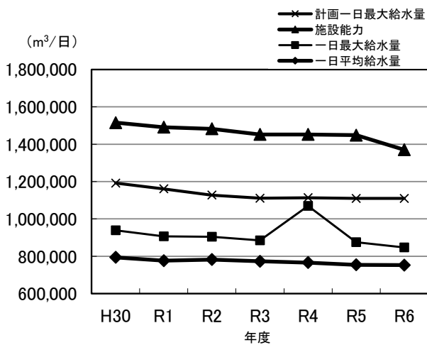
一日当たり給水量の推移
