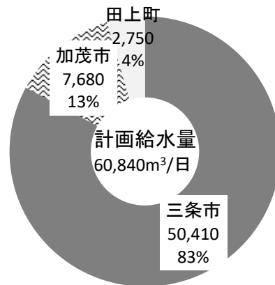
三条地域水道用水供給企業団 構成団体の計画給水量
