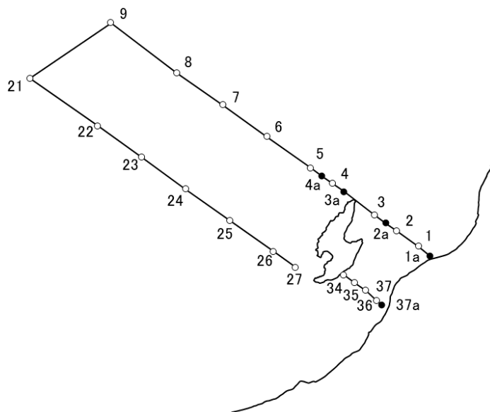
図1 沿岸沖合定線
