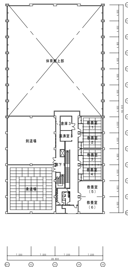
職員会館 2階平面図
