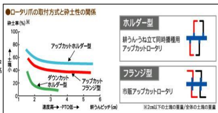
図2 ロータリ爪の取付方式と砕土性の関係 (農研機構中央農研・北陸水田輪作研究チーム)
