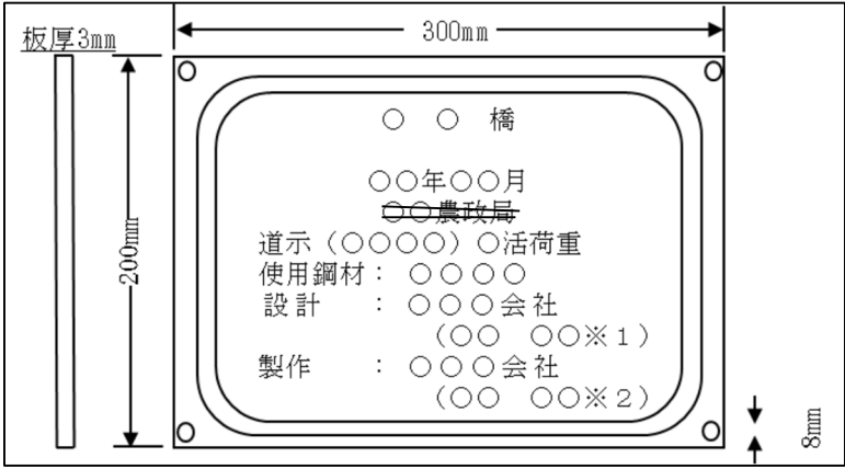
※1 管理技術者氏名、※2 監理技術者氏名 図10-1-1 銘板の寸法及び記載事項
