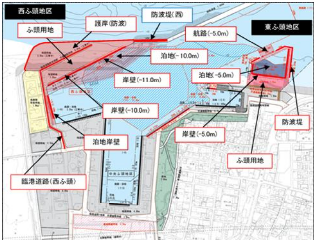
姫川港 港湾改修平面図
