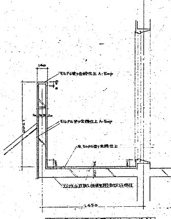
最上階手摺断面 (PHが省略)
