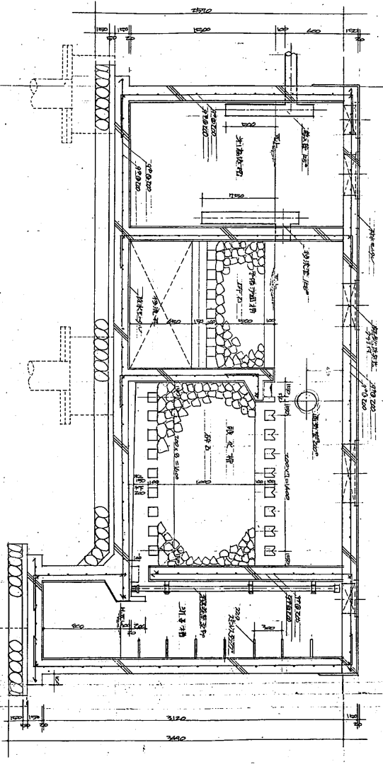
A-A断面图 1:20
