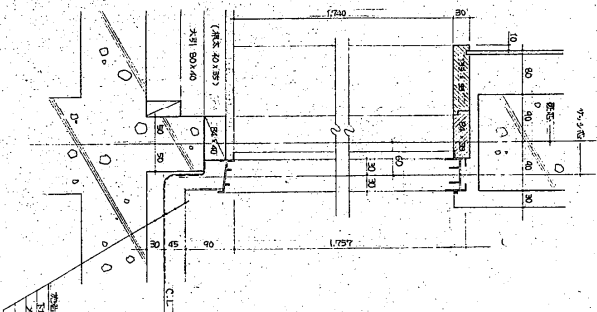
图 S-1-5 无望入口断面详细图
