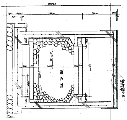
B-B断面图 1:20
