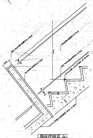
階段詳細図 1/20
