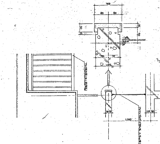
バルコニー設置時除却スクリン 詳細図 S-1:2b
