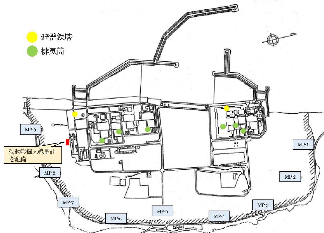
図10 構内配置図
