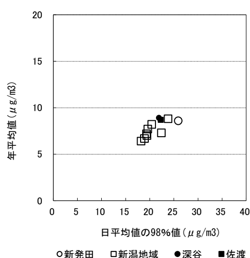
図 1-3-1-10 微小粒子状物質(PM 2.5 )
