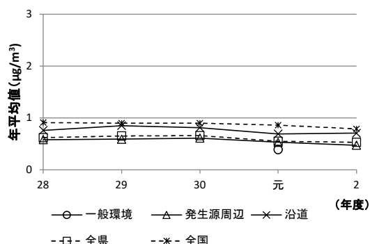
図 1-3-3-4 ベンゼン年平均値の経年変化
