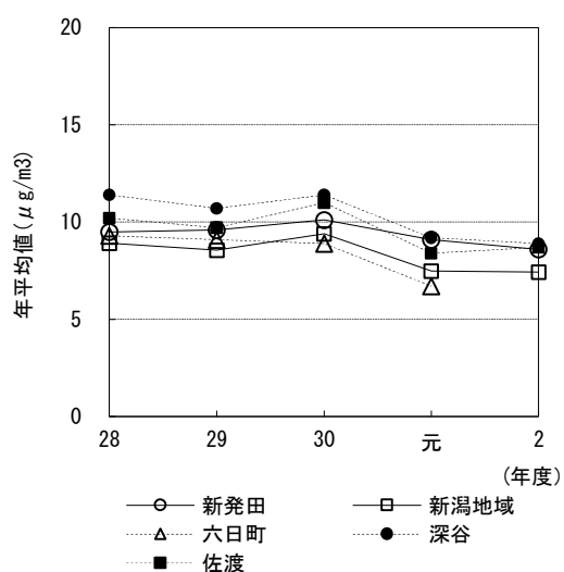
図 1-3-1-9 微小粒子状物質(PM 2.5 )
