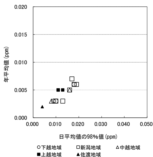
図1-3-1-4 二酸化窒素(NO 2 )日平均値の年間98%値と年平均値の分布
