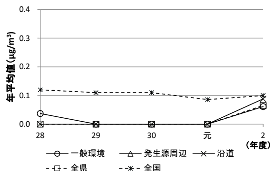
図 1-3-3-2 テトラクロロエチレン年平均値の経年変化
