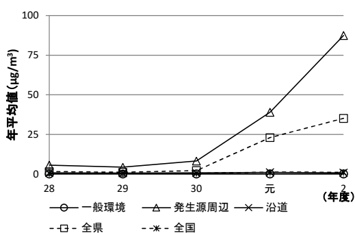
図 1-3-3-3 トリクロロエチレン年平均値の経年変化
