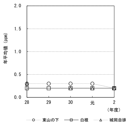
図 1-3-2-3 光化学オキシダント(O x )環境基準超過時間割合の経年変化
