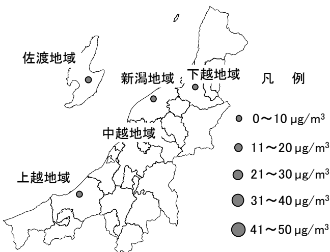
図 1-3-1-16 微小粒子状物質(PM2.5)年平均值の地域平均
