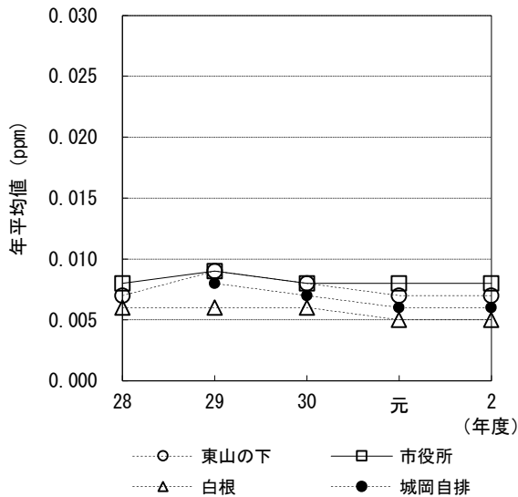
図 1-3-2-1 二酸化窒素(NO 2 )年平均値の経年変化
