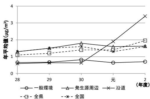
図 1-3-3-1 ジクロロメタン年平均値の経年変化
