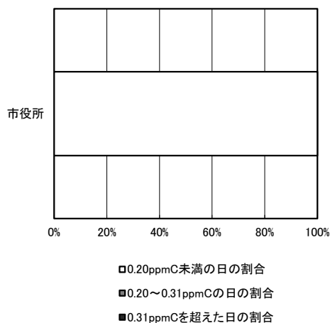
図1-3-2-4 非メタン炭化水素午前6～9時3時間平均値の指針値との対応
