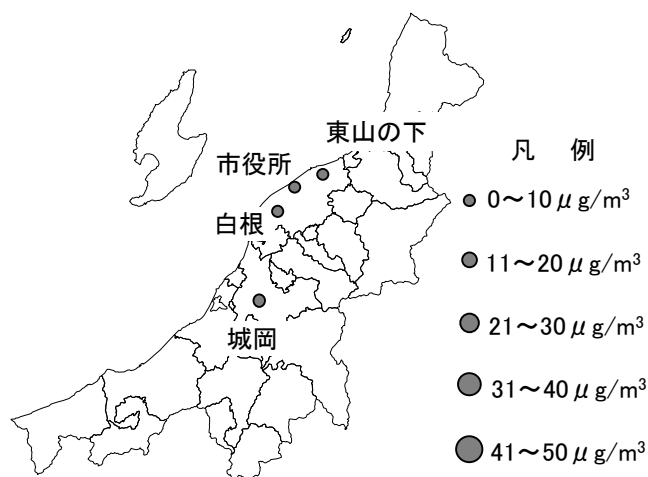
図 1-3-2-10 微小粒子状物質(PM2.5)年平均值
