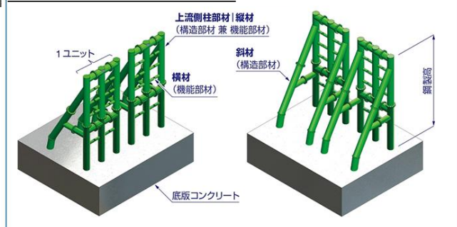
鋼製スリットイメージ
