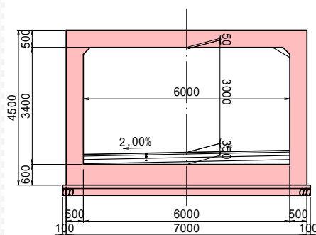
横断函渠 断面図
