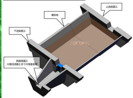
土砂溜め立体イメージ
